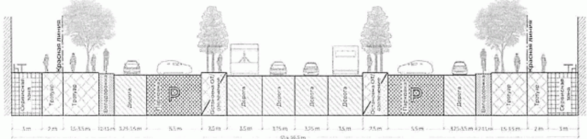
Магистральная улица тип 2
