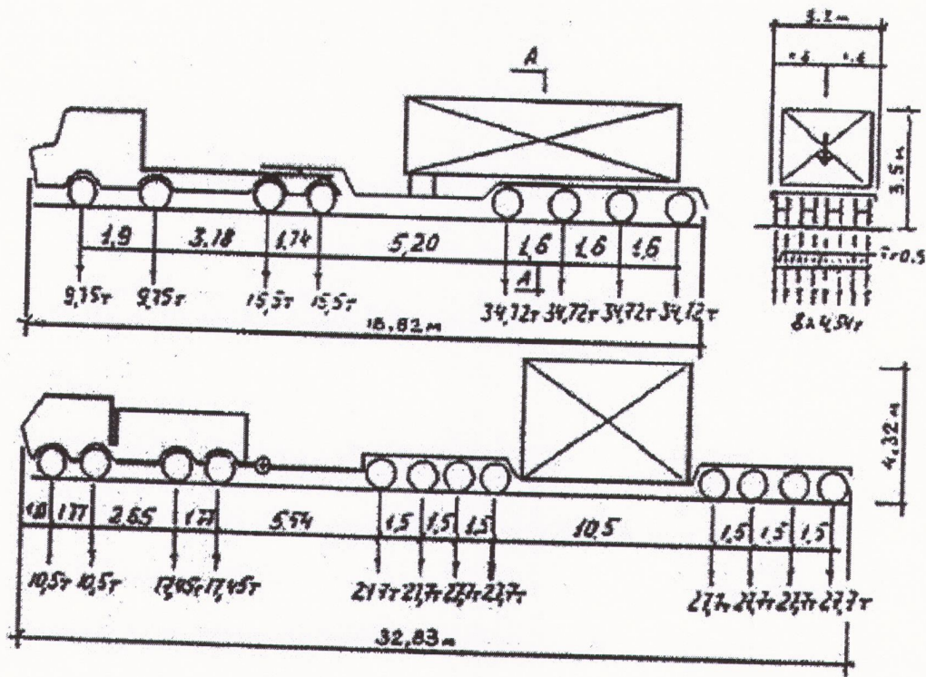
Схема автопоезда
